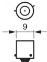
BAX9s
