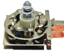
DIODISILTA
